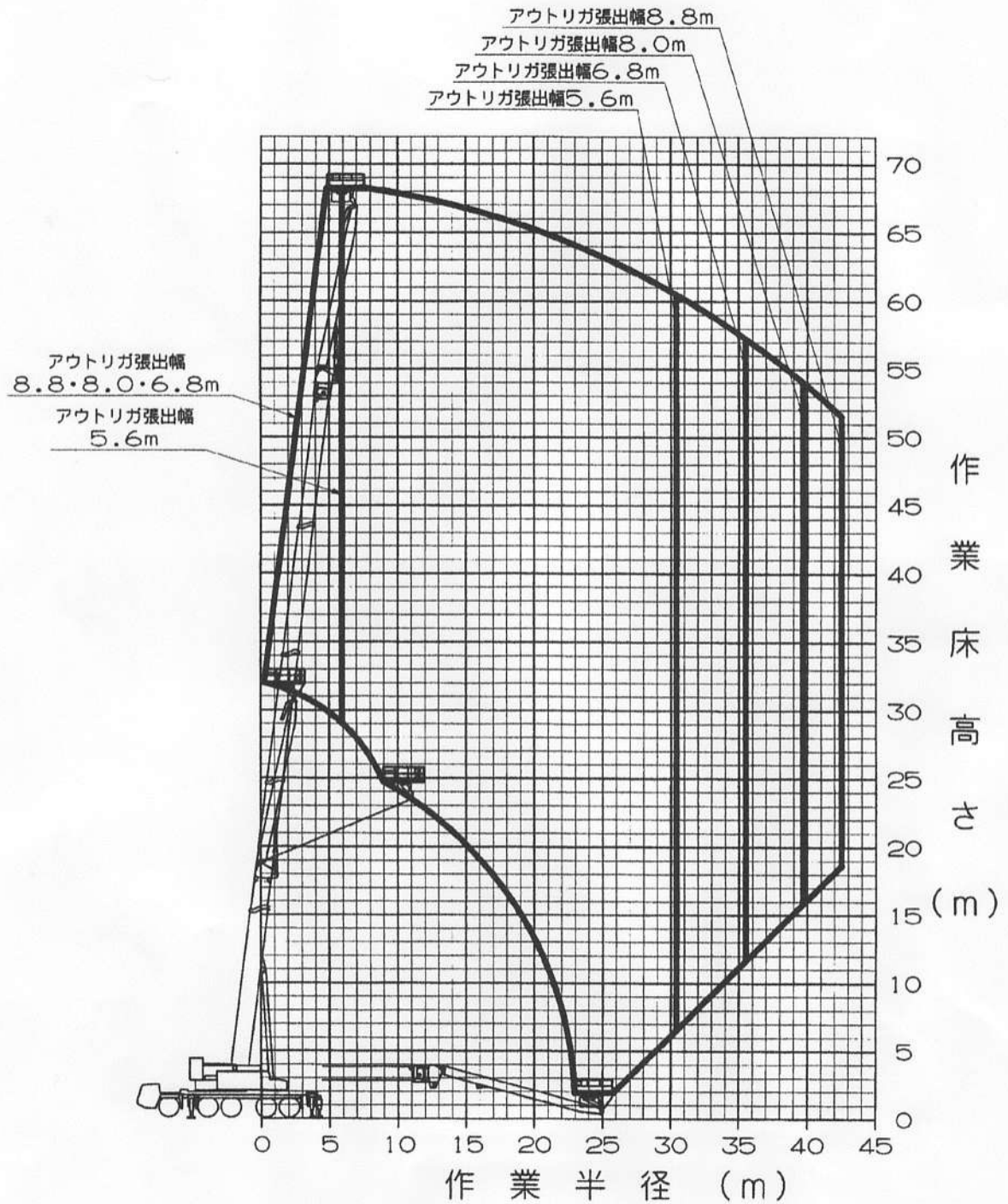
4-6 作業範囲図6 [デッキ最大積載荷重1.0t]
