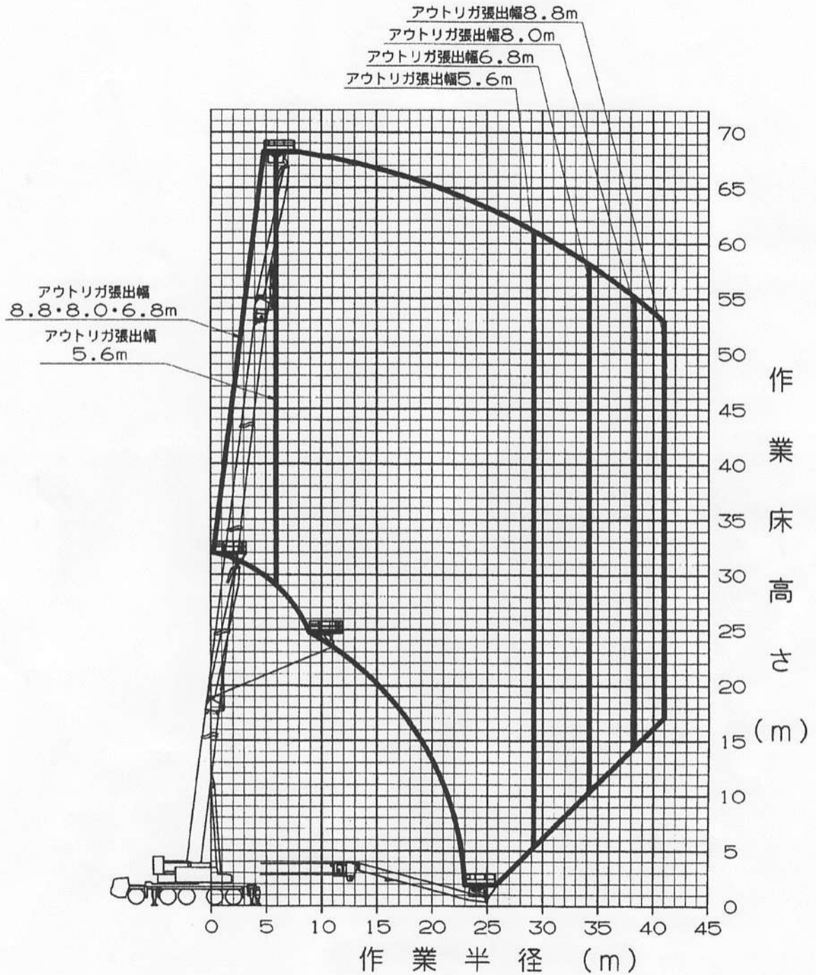
4-5 作業範囲図5 [デッキ最大積載荷重1.5t]
